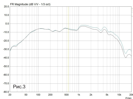
АЧХ с фильтром первого порядка.
