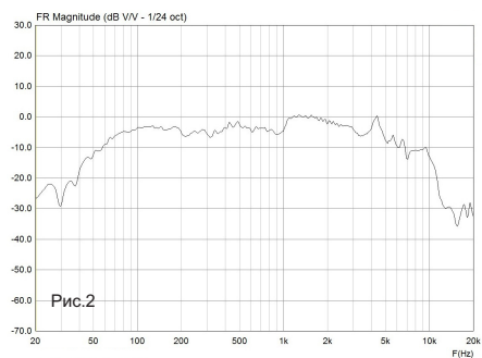
мв1602.1.4 АЧХ сглаживание 1/24
