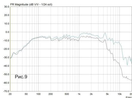
АЧХ с фильтром второго порядка.
