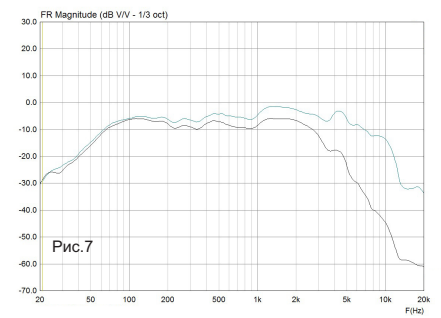
АЧХ с фильтром второго порядка.
